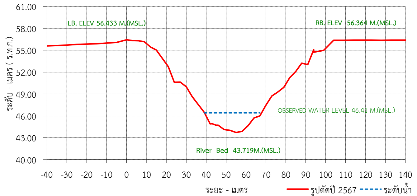
รูปตัดขวางลำน้ำ ปีน้ำ 2567 สถานี Y.33 แม่น้ำยม อ.ศรีสำโรง จ.สุโขทัย
